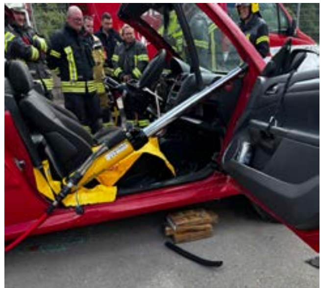
Vornahme eines hydraulischen Stempels
