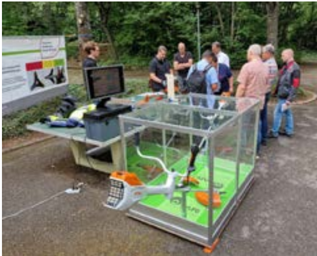
Ein Simulationsgerät vermittelt Vibrationen praxisnah. Foto: SVLFG
